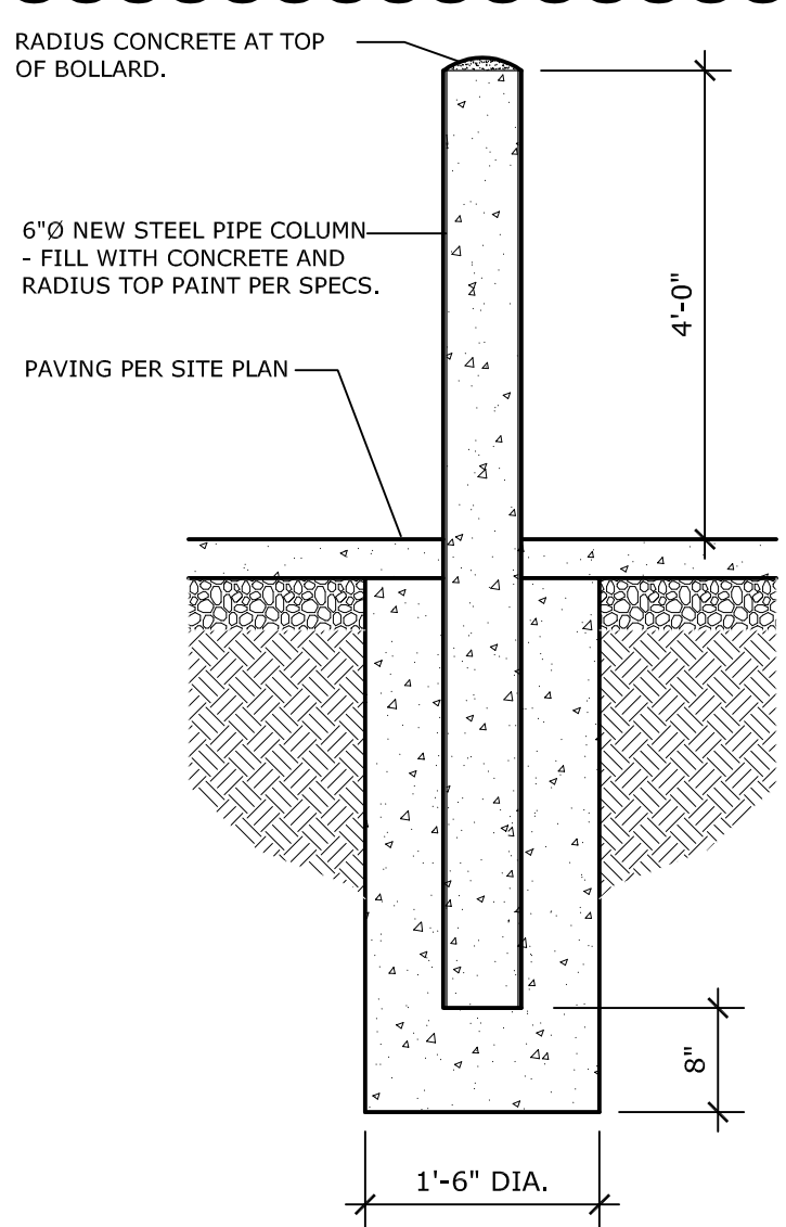
5P BOLLARD SECTION AS102 scale: 3/4" = 1'-0"
